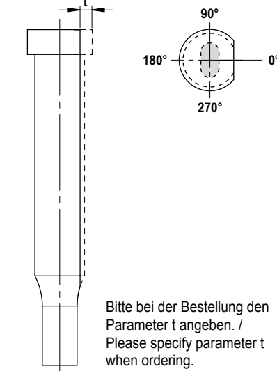
Verdrehsicherung / rotation prevention Type V3
