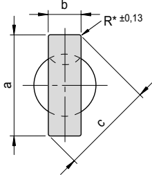
Typ / Type L
