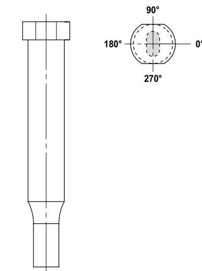
Verdrehsicherung / rotation prevention Type V2
