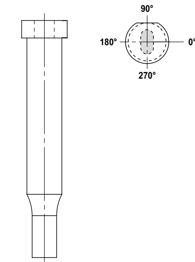
Verdrehsicherung / rotation prevention Type V1
