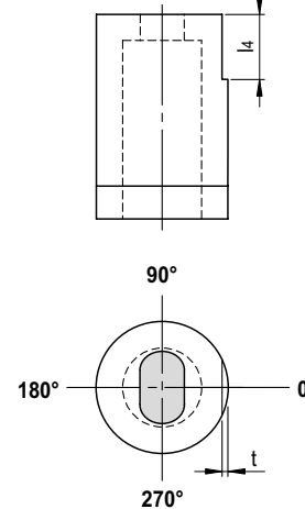
Verdrehsicherung / Rotation prevention Type V7
