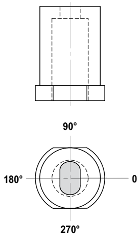
Verdrehsicherung Typ V5 Rotation prevention Type V5
