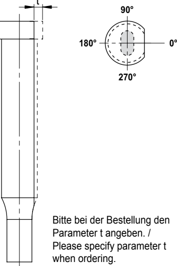
Verdrehsicherung Typ V3 Rotation prevention Type V3
