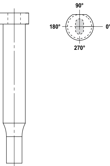
Verdrehsicherung Typ V1 Rotation prevention Type V1
