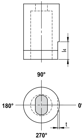
Verdrehsicherung Typ V6 Rotation prevention Type V6
