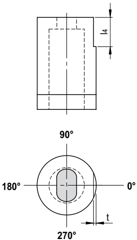
Verdrehsicherung Typ V7 Rotation prevention Type V7
