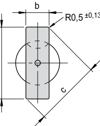
Typ / Type H
