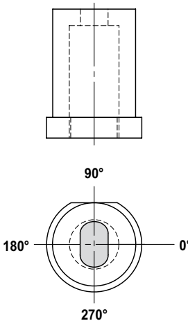
Verdrehsicherung Typ V4 Rotation prevention Type V4
