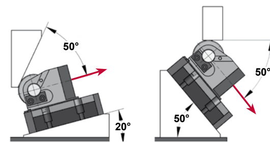
Max. Schrägeinbau / Max. working angle
